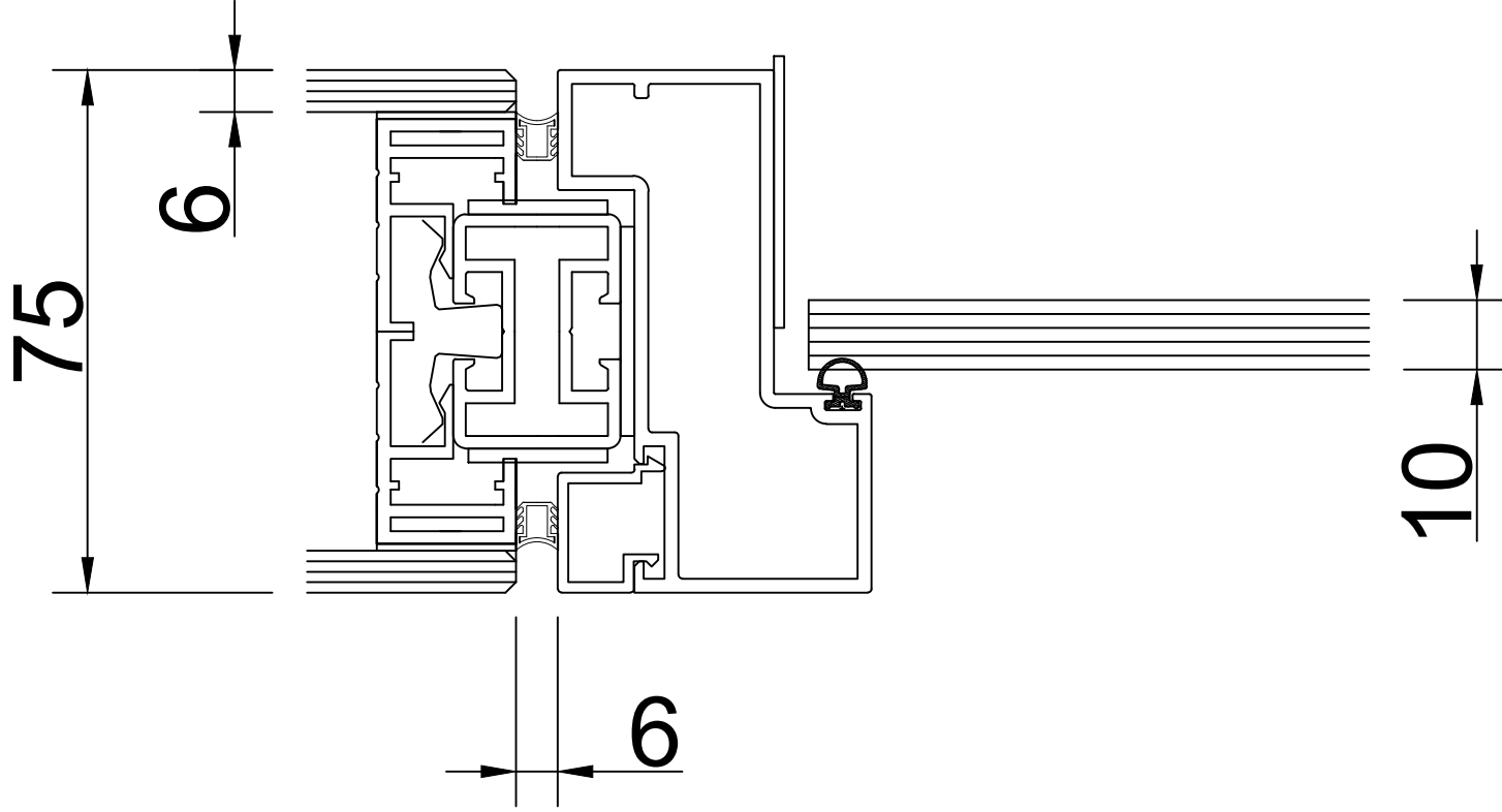
CAM - KAPI BİRLEŞİMİ
