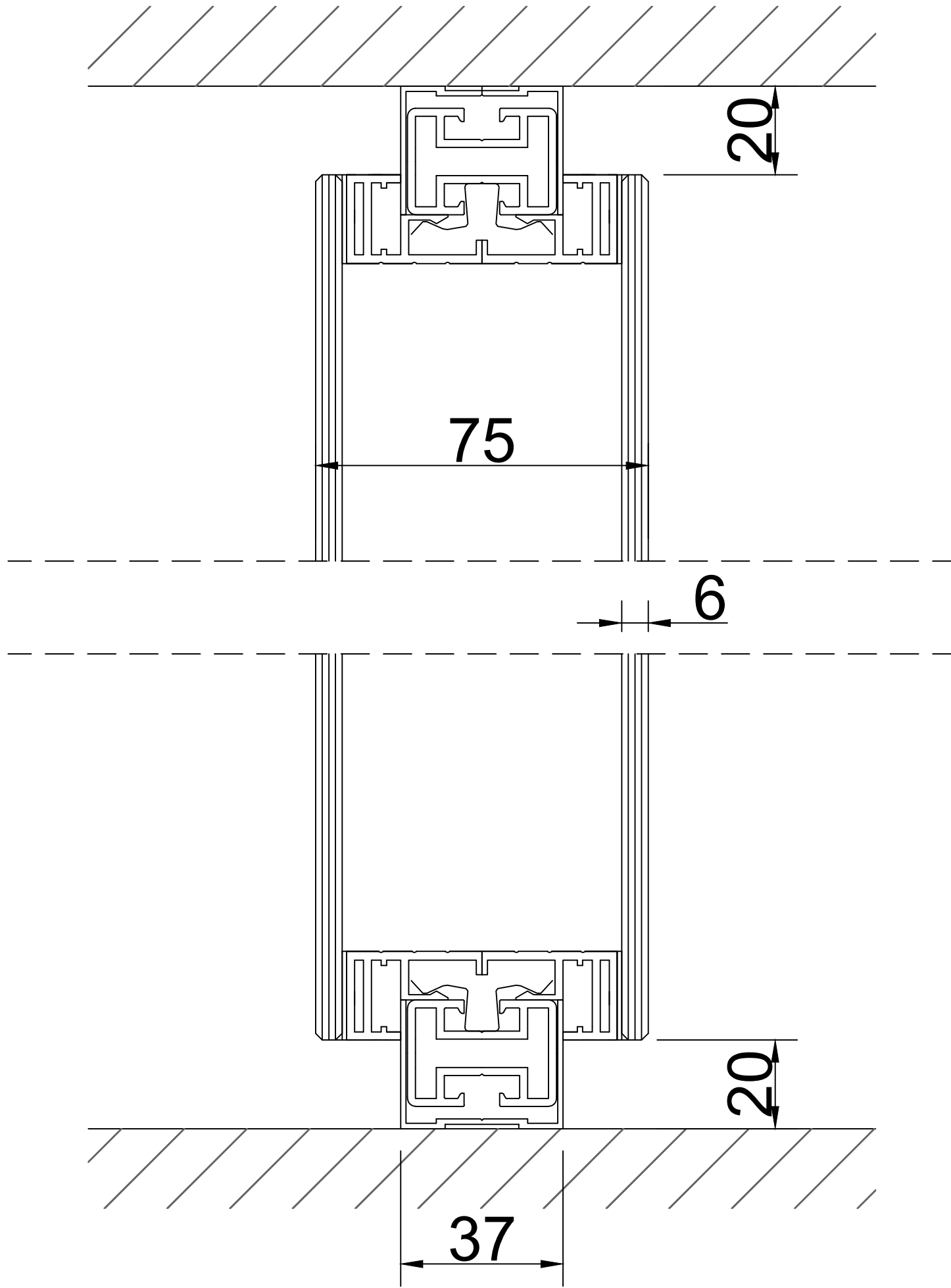
SİSTEM KESİTİ
