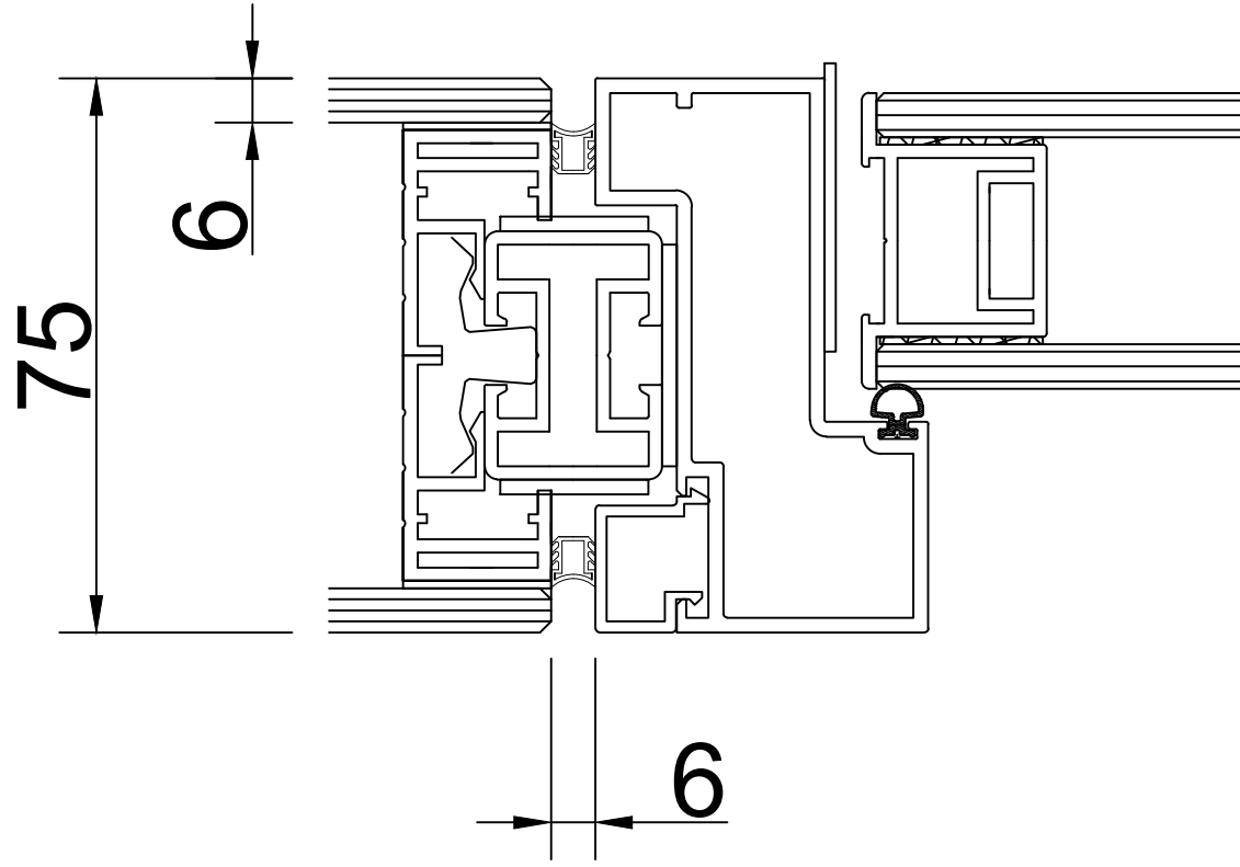
CAM - ÇİFT CAMLI KAPI BİRLEŞİMİ
