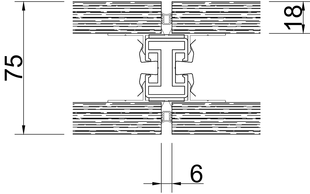
AHŞAP - AHŞAP BİRLEŞİMİ
