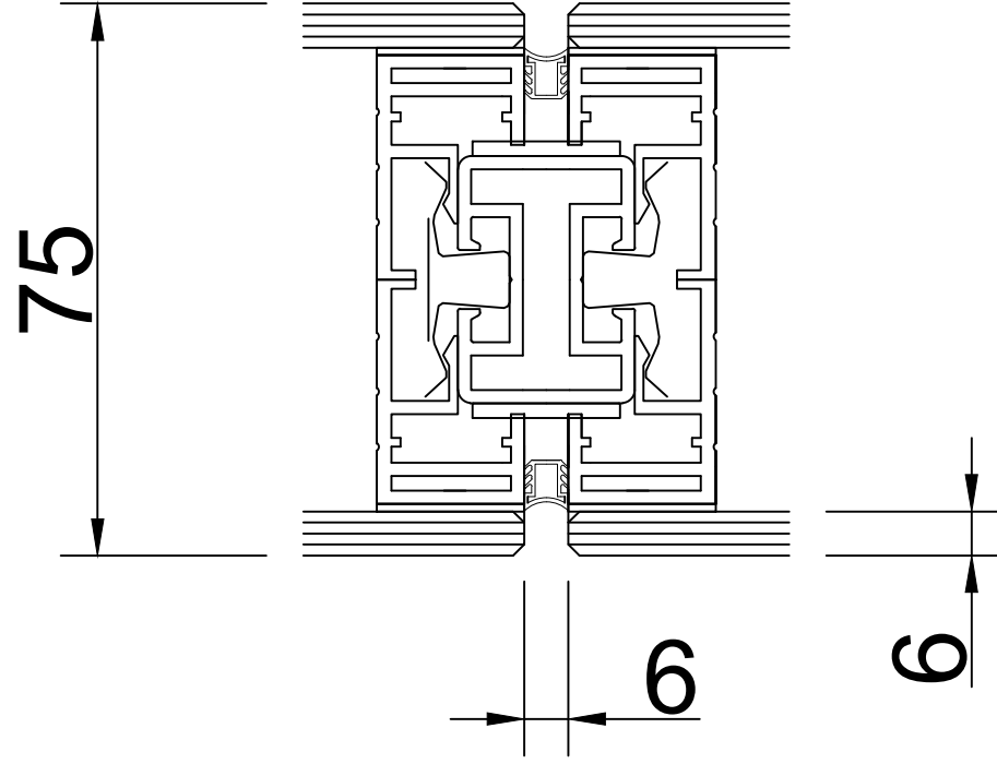
CAM - CAM BİRLEŞİMİ
