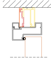
ahşap kapı kasası tavan kesiti
