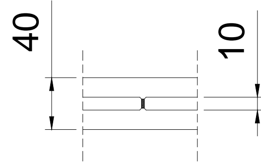
2mm VHB bant ile cam cama birleşim
