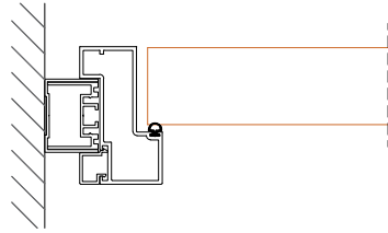
duvar - ahşap kapı kasası birleşim
