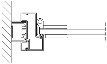
duvar - cam kapı kasası birleşim
