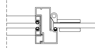
cam - kapı kasası birleşim
