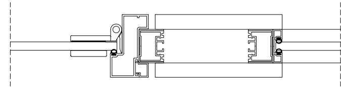
kapı kasası - dolu - cam birleşim
