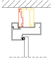
cam kapı kasası tavan kesiti
